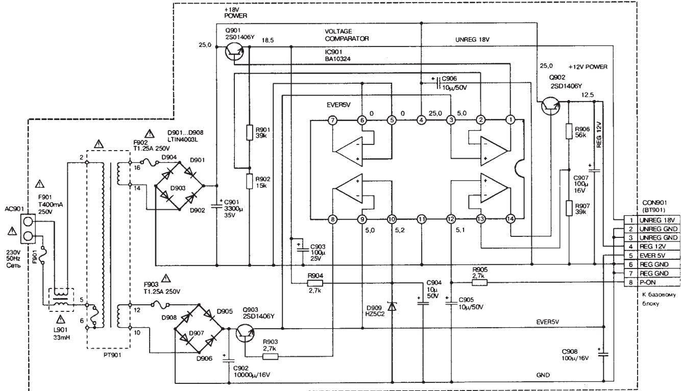
Рис. 2.4. Принципиальная схема источника питания видеоплеера HV-SX1.
